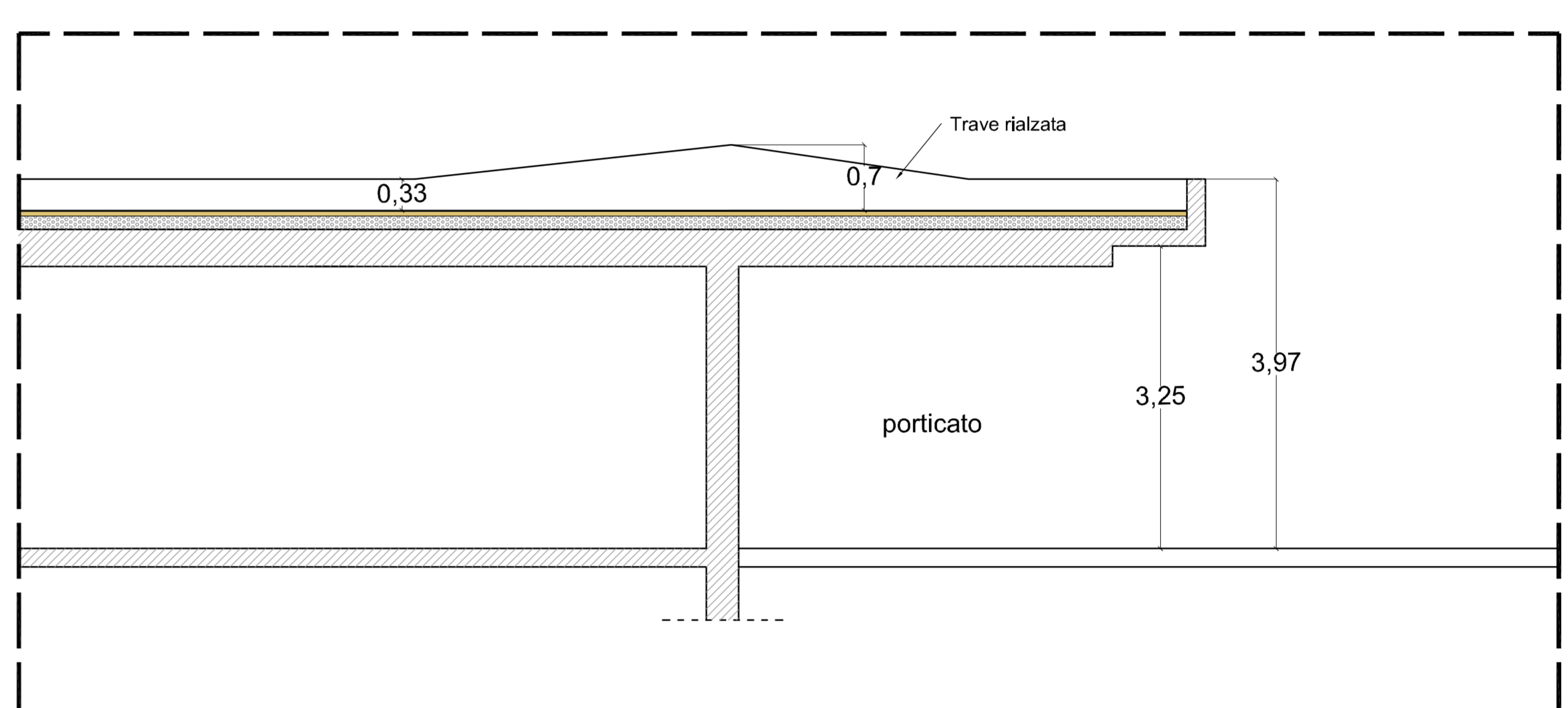
PROFILO MURETTO GIUNTO STRUTTURALE 1 - scala 1:50
