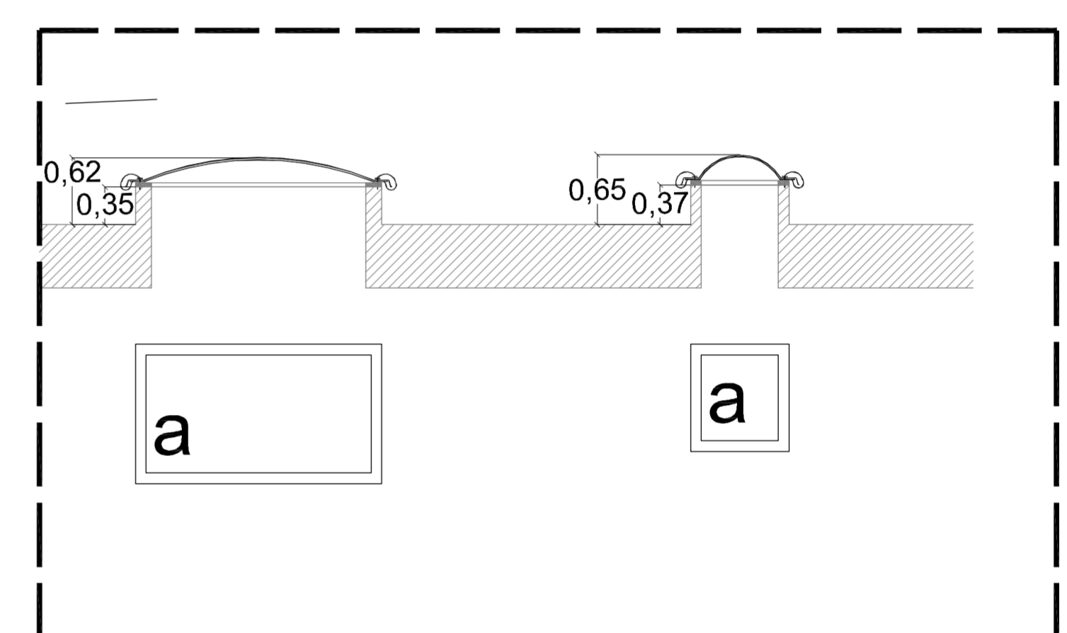
DETTAGLIO CUPOLINI TIPO- scala 1:50
