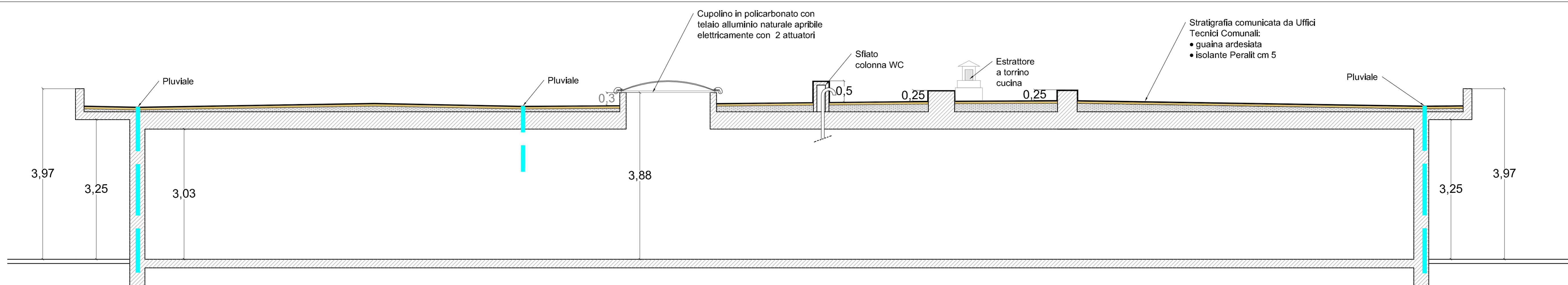
SEZIONE A-A' - scala 1:50
